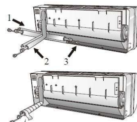
Łączenie rurki przyłączeniowej
